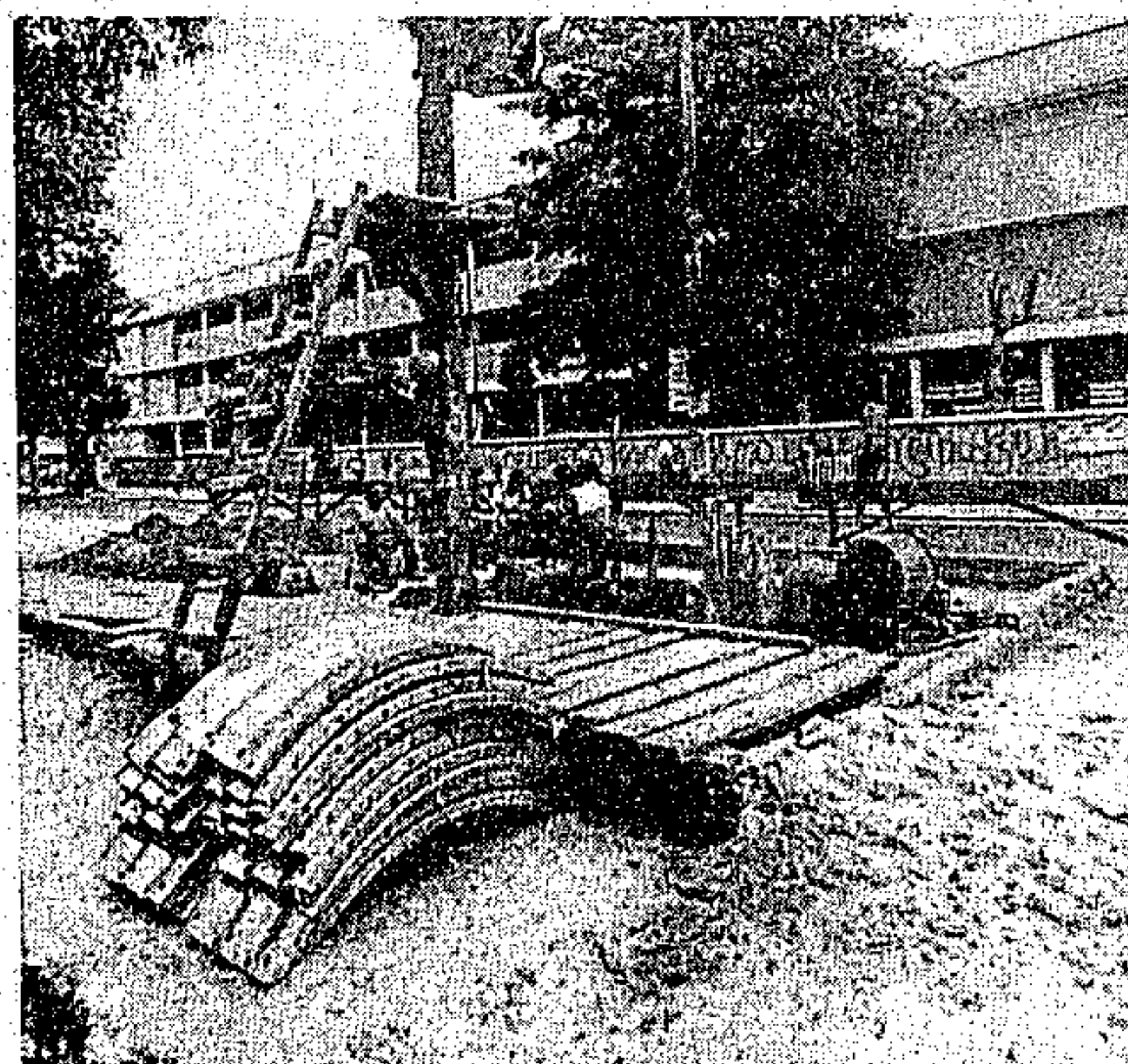
O Tunnel Liner da Sub-Adutora do 4º Setor, quase pronto.
