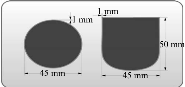
Figura 049 – Base do distintivo emborrachado de cursos militares de carreira (bolso) (medidas).
